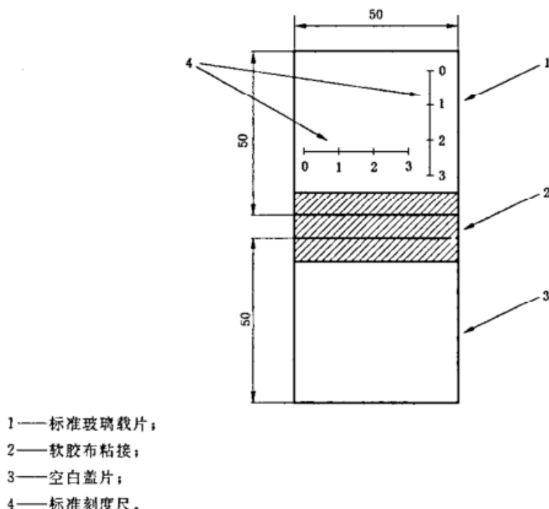
图3 载片装置
